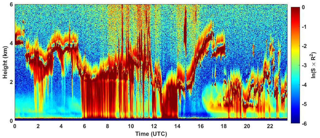
2020-02-14 RCS quick look CHM15k - ILVA LIDAR1 DIREZIONE
