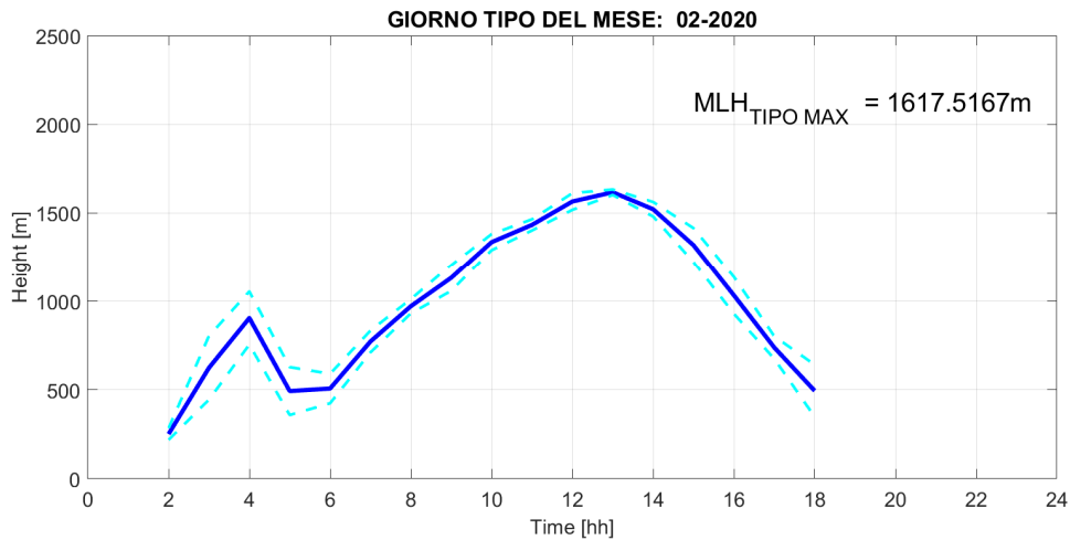
Fig. 2: Giorno tipo del parametro Mixing Layer Height nel mese di FEBBRAIO 2020, rappresentato mediante media oraria (linea blu continua) e deviazione standard (linee celesti tratteggiate).
