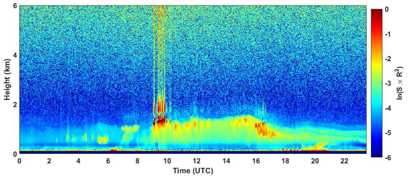
2020-02-16 RCS quick look CHM15k - ILVA LIDAR1 DIREZIONE
