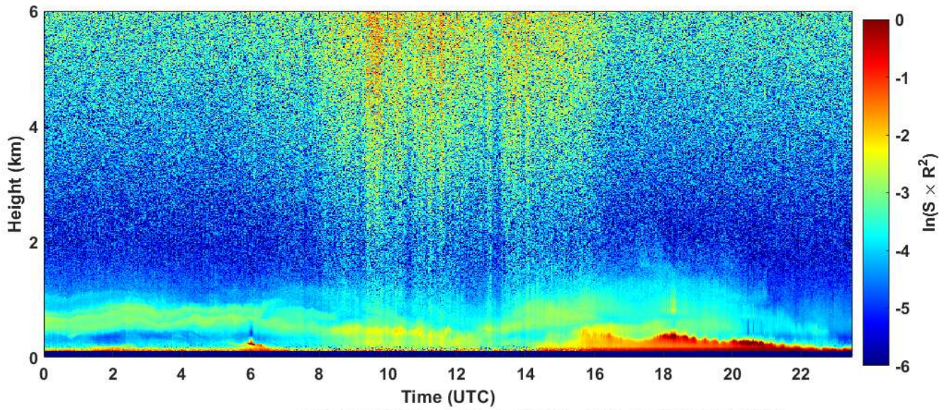
2020-02-26 RCS quick look CHM15k - ILVA LIDAR1 DIREZIONE
