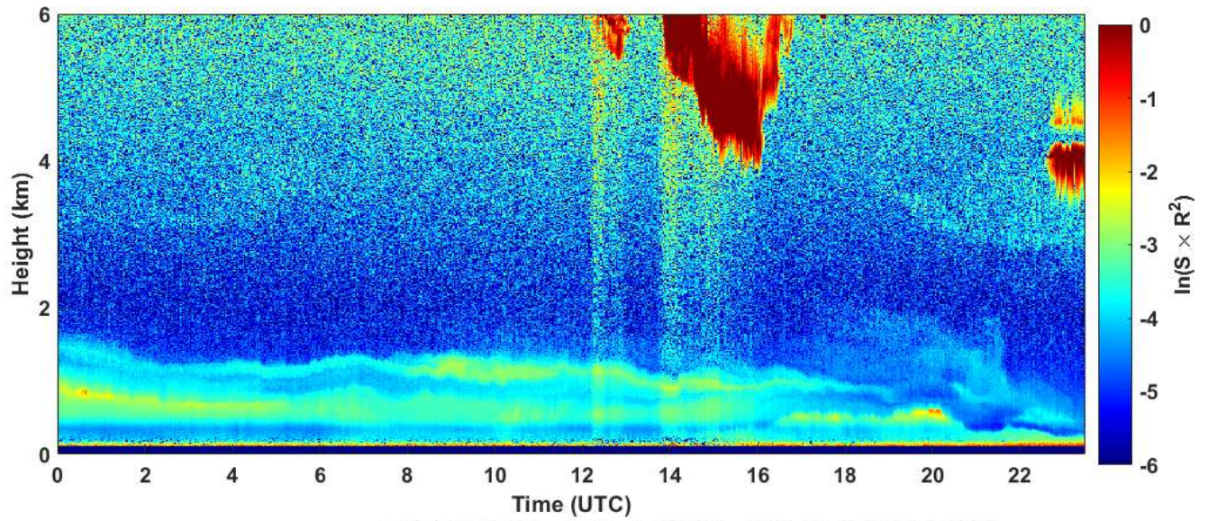
2020-02-10 RCS quick look CHM15k - ILVA LIDAR1 DIREZIONE
