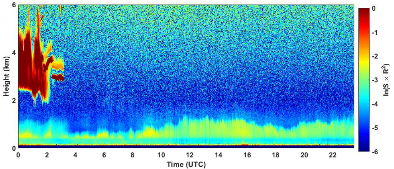
2020-01-02 RCS quick look CHM15k - ILVA LIDAR1 DIREZIONE
