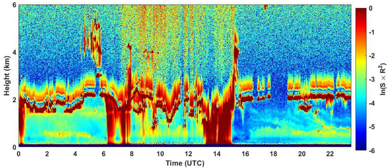
2020-01-14 RCS quick look CHM15k - ILVA LIDAR1 DIREZIONE
