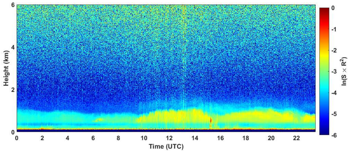
2020-01-22 RCS quick look CHM15k - ILVA LIDAR1 DIREZIONE
