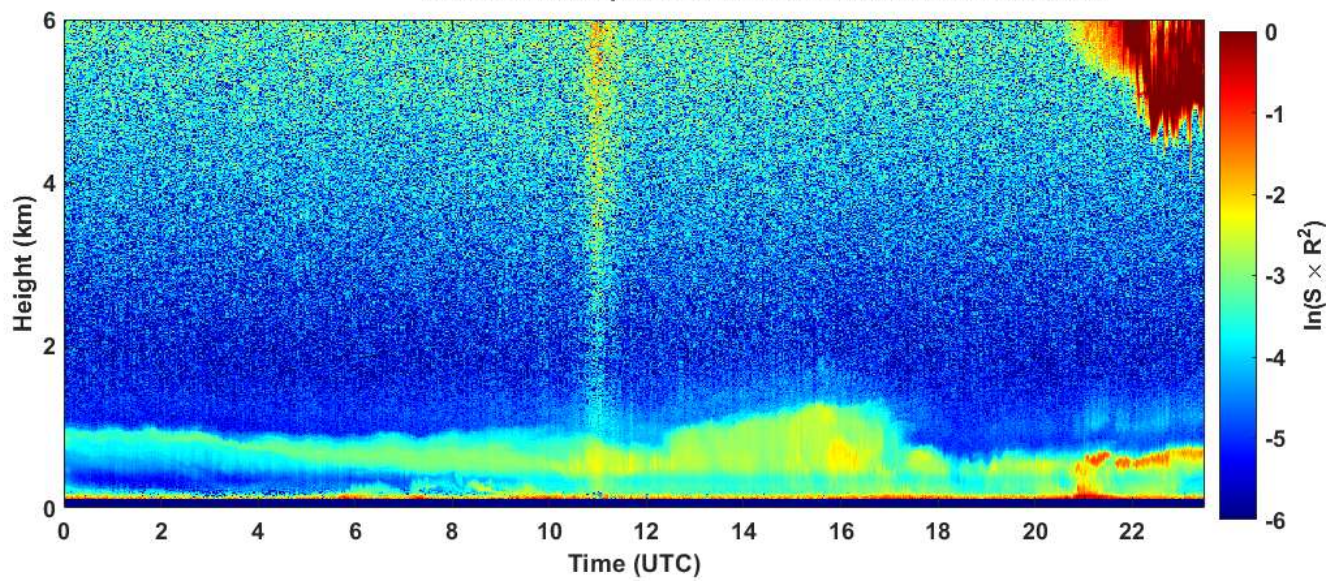
2020-01-10 RCS quick look CHM15k - ILVA LIDAR1 DIREZIONE
