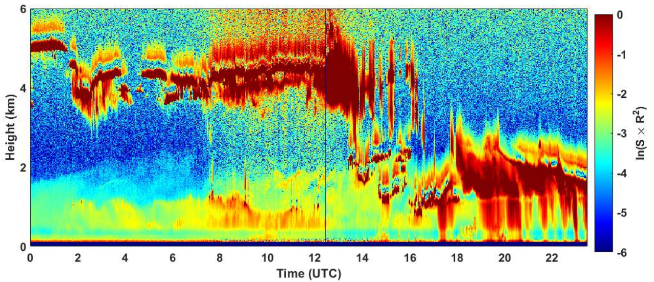
2020-01-12 RCS quick look CHM15k - ILVA LIDAR1 DIREZIONE
