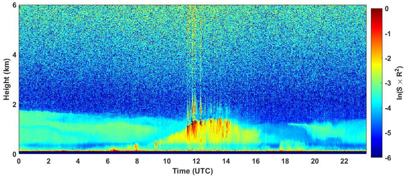
2020-01-16 RCS quick look CHM15k - ILVA LIDAR1 DIREZIONE
