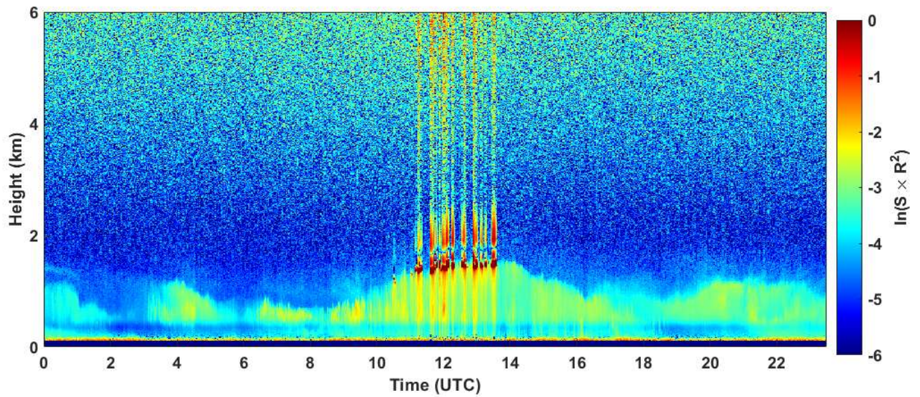
2020-01-08 RCS quick look CHM15k - ILVA LIDAR1 DIREZIONE
