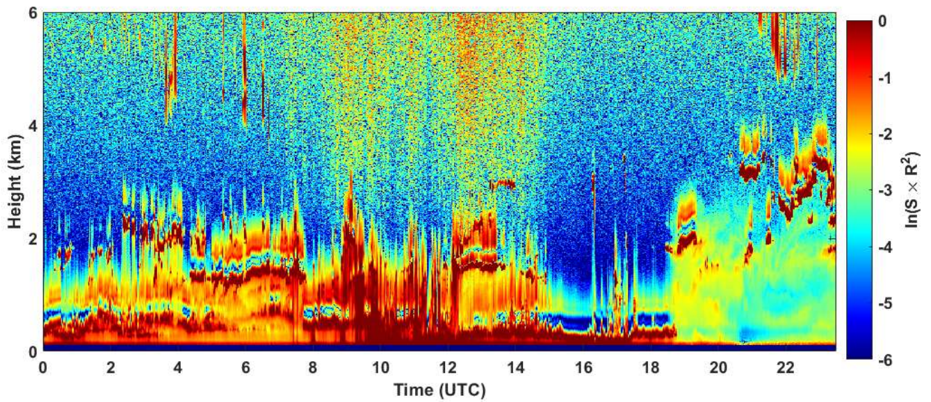
2020-01-26 RCS quick look CHM15k - ILVA LIDAR1 DIREZIONE
