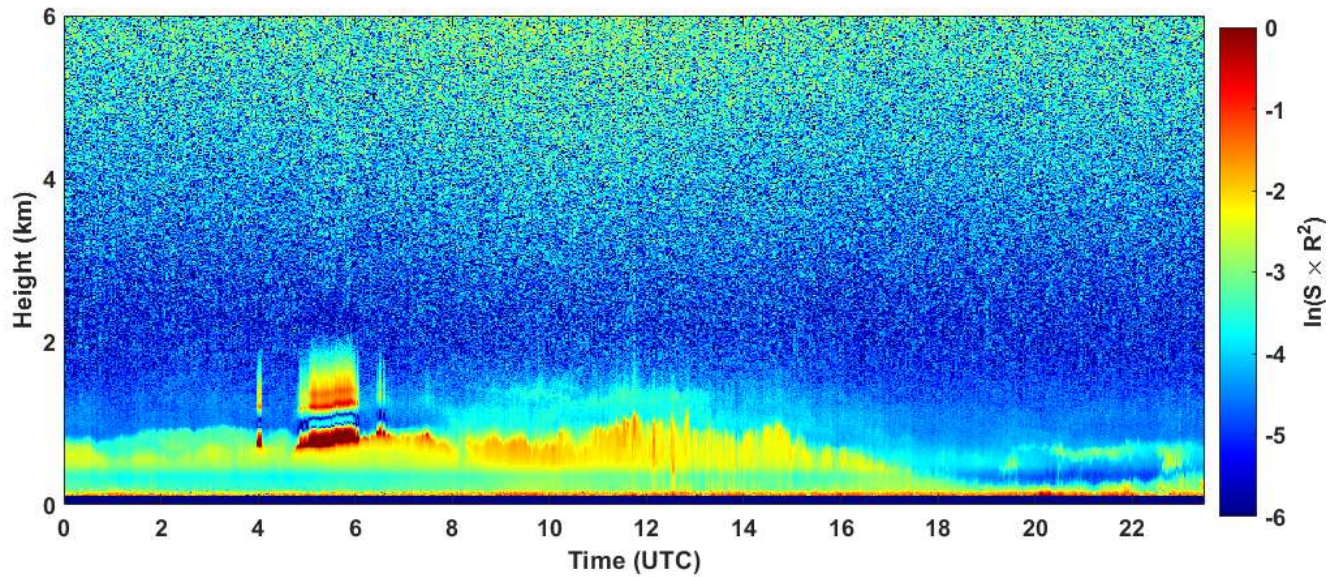
2020-01-24 RCS quick look CHM15k - ILVA LIDAR1 DIREZIONE
