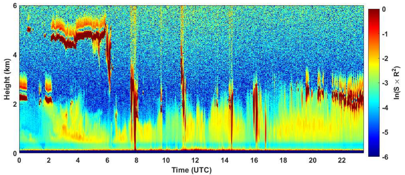
2020-01-06 RCS quick look CHM15k - ILVA LIDAR1 DIREZIONE
