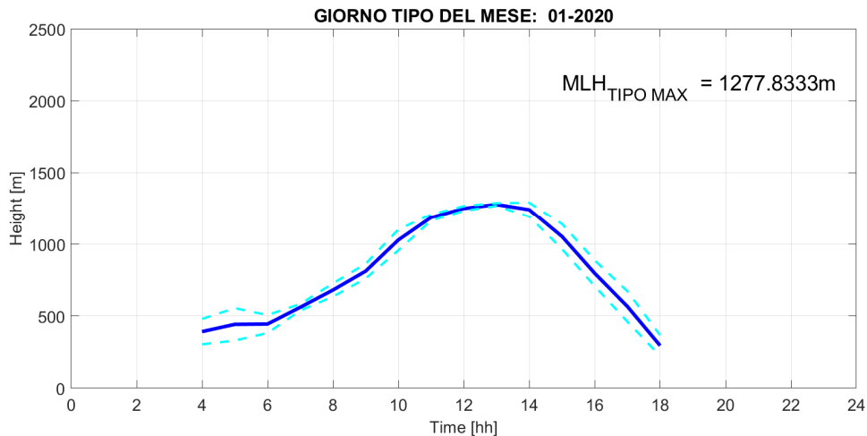
Fig. 2: Giorno tipo del parametro Mixing Layer Height nel mese di GENNAIO 2020, rappresentato mediante media oraria (linea blu continua) e deviazione standard (linee celesti tratteggiate).
