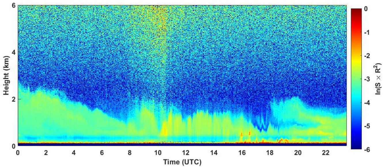
2020-01-30 RCS quick look CHM15k - ILVA LIDAR1 DIREZIONE
