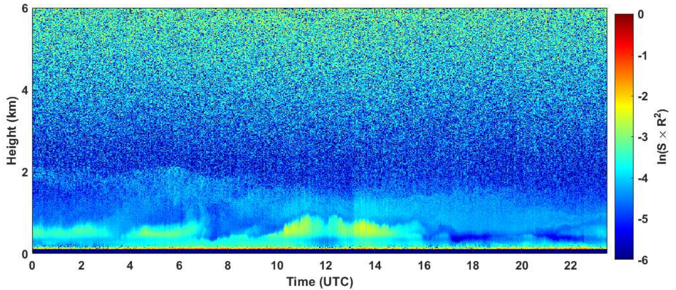
2020-01-04 RCS quick look CHM15k - ILVA LIDAR1 DIREZIONE
