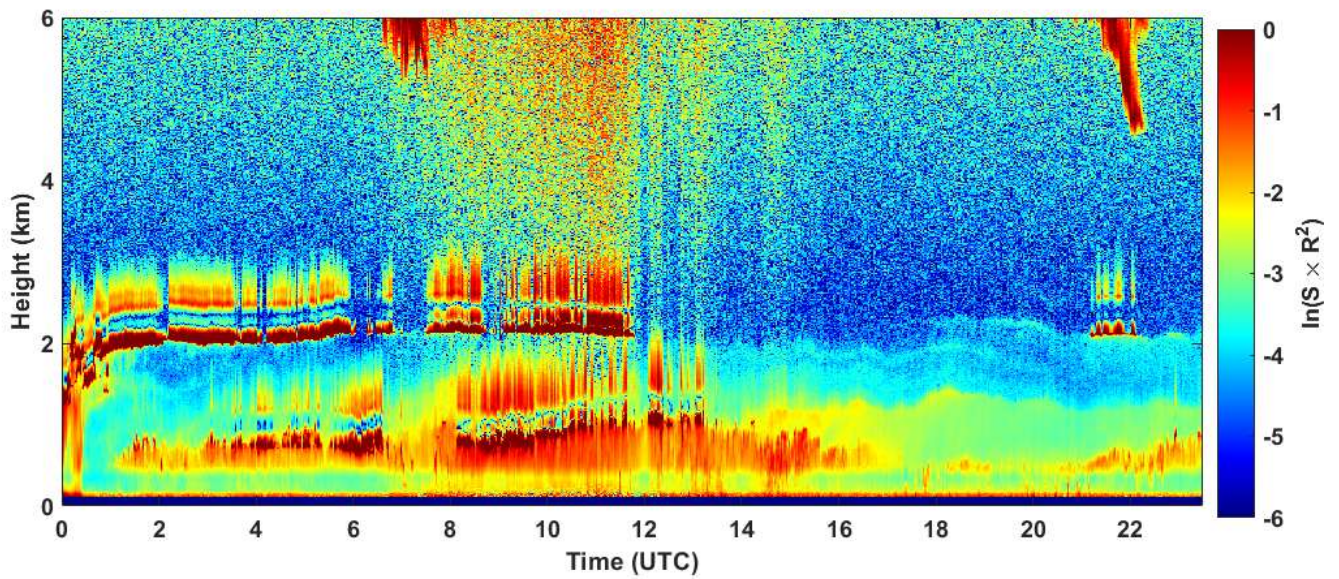
2020-01-20 RCS quick look CHM15k - ILVA LIDAR1 DIREZIONE
