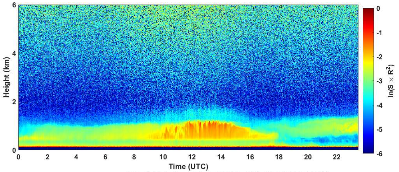
2020-01-18 RCS quick look CHM15k - ILVA LIDAR1 DIREZIONE
