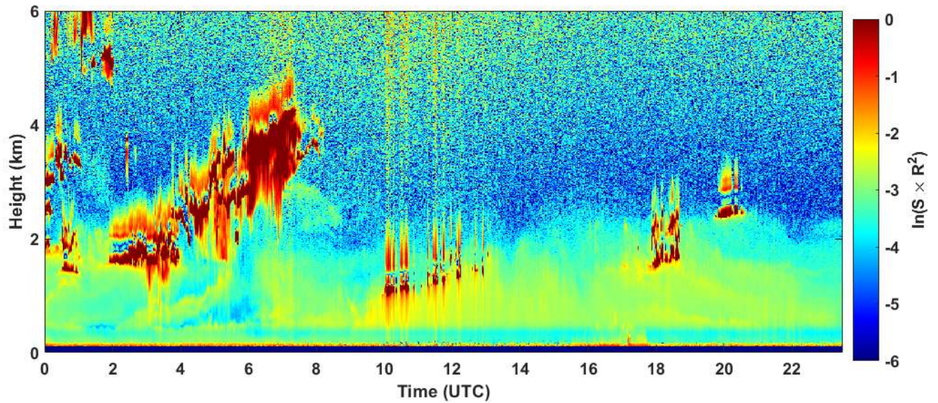
2020-01-28 RCS quick look CHM15k - ILVA LIDAR1 DIREZIONE
