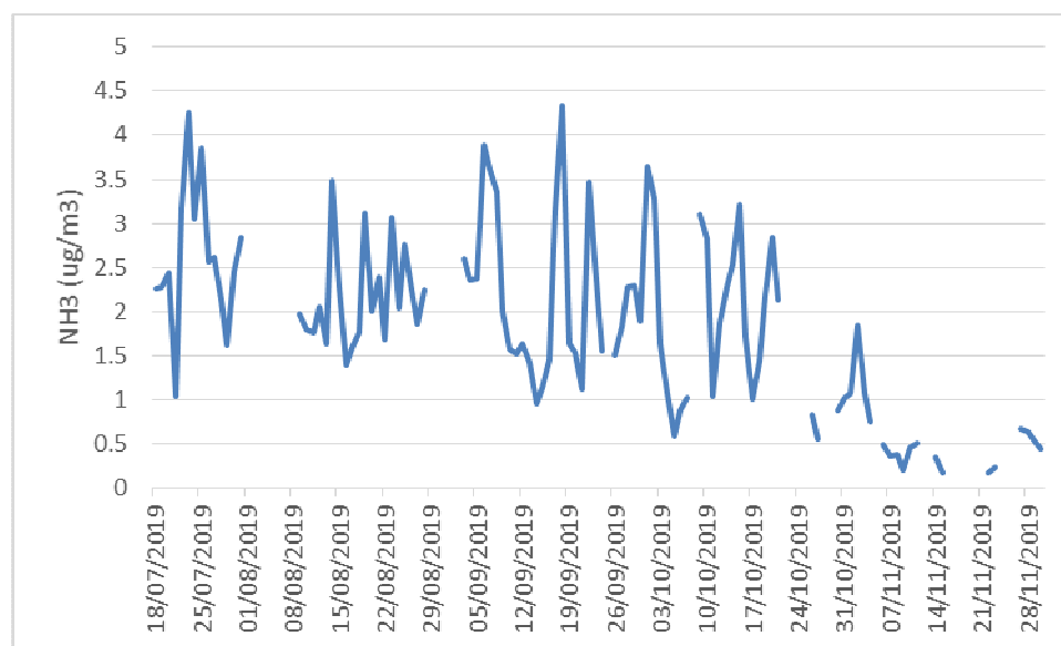
Figura 9. NH 3 : media giornaliera
