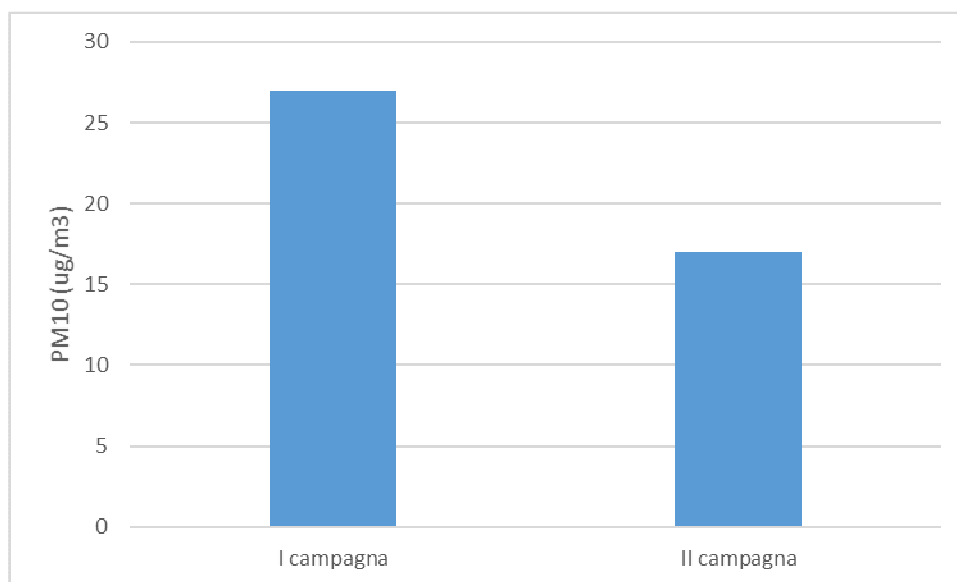
Figura 10. PM10: confronto tra prima e seconda campagna di monitoraggio
