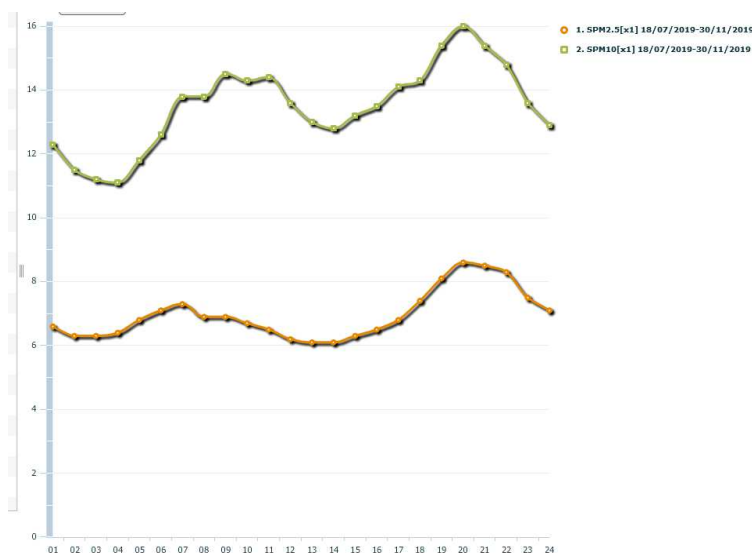
Figura 4a. PMx: giorno tipo
