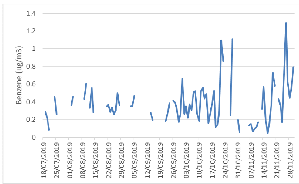
Figura 7. Benzene: media giornaliera
