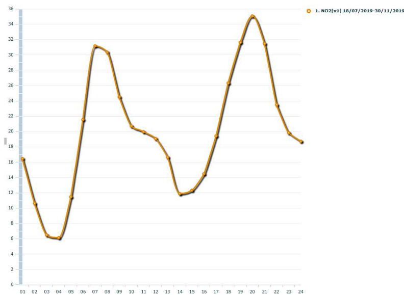
Figura 5c. NO 2 : giorno tipo
