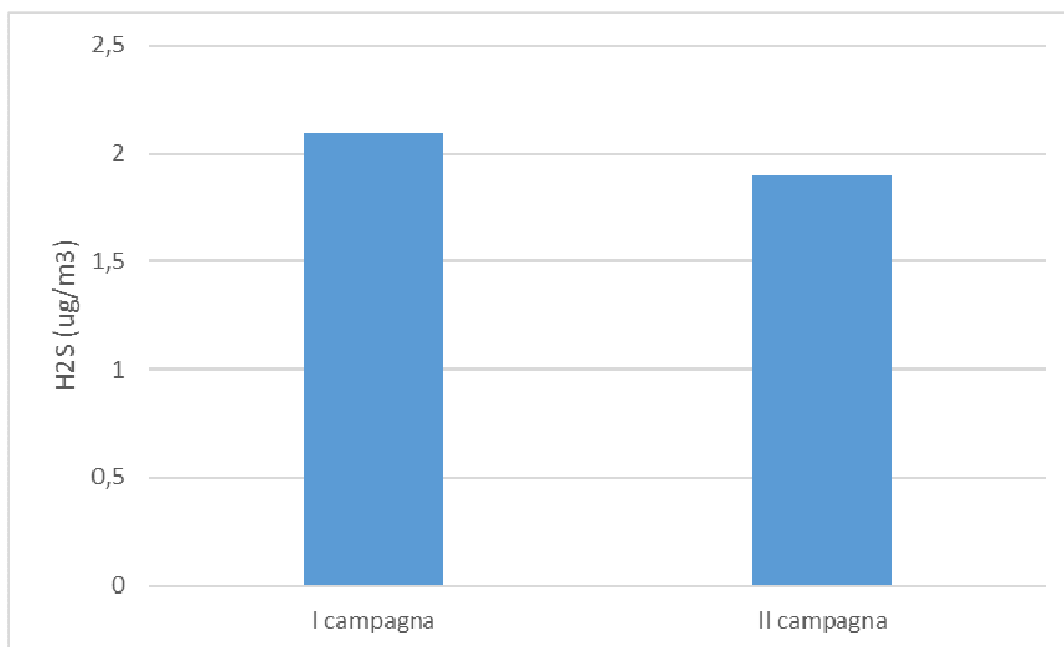
Figura 14. H2S: confronto tra prima e seconda campagna di monitoraggio
