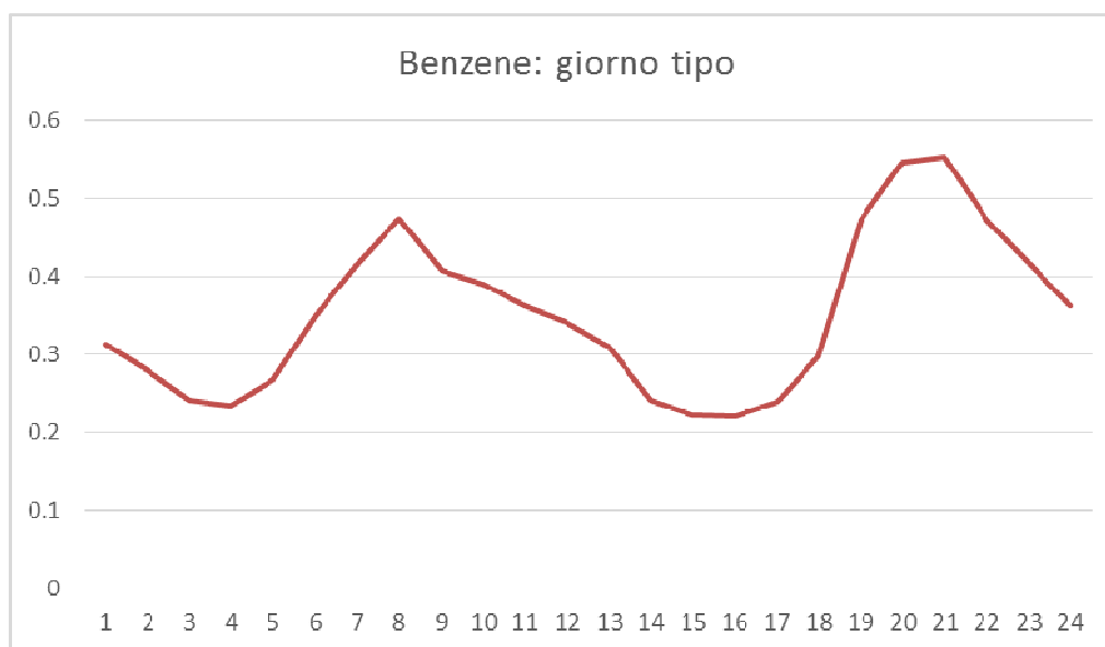
Figura 5b. Benzene: giorno tipo
