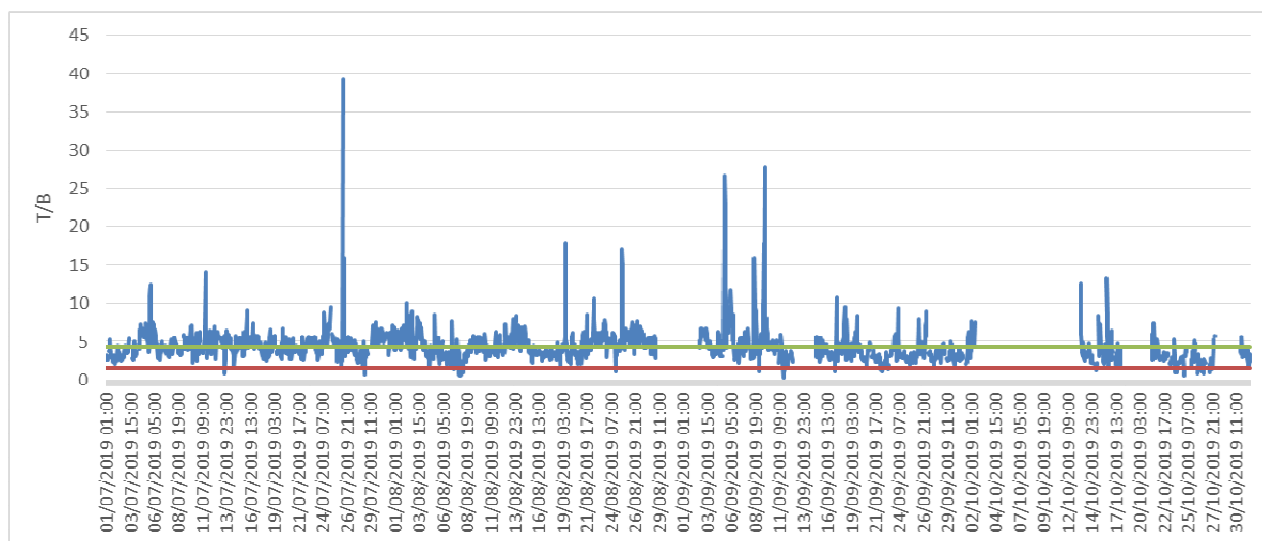
Figura 5c. Rapporto Toluene/Benzene
