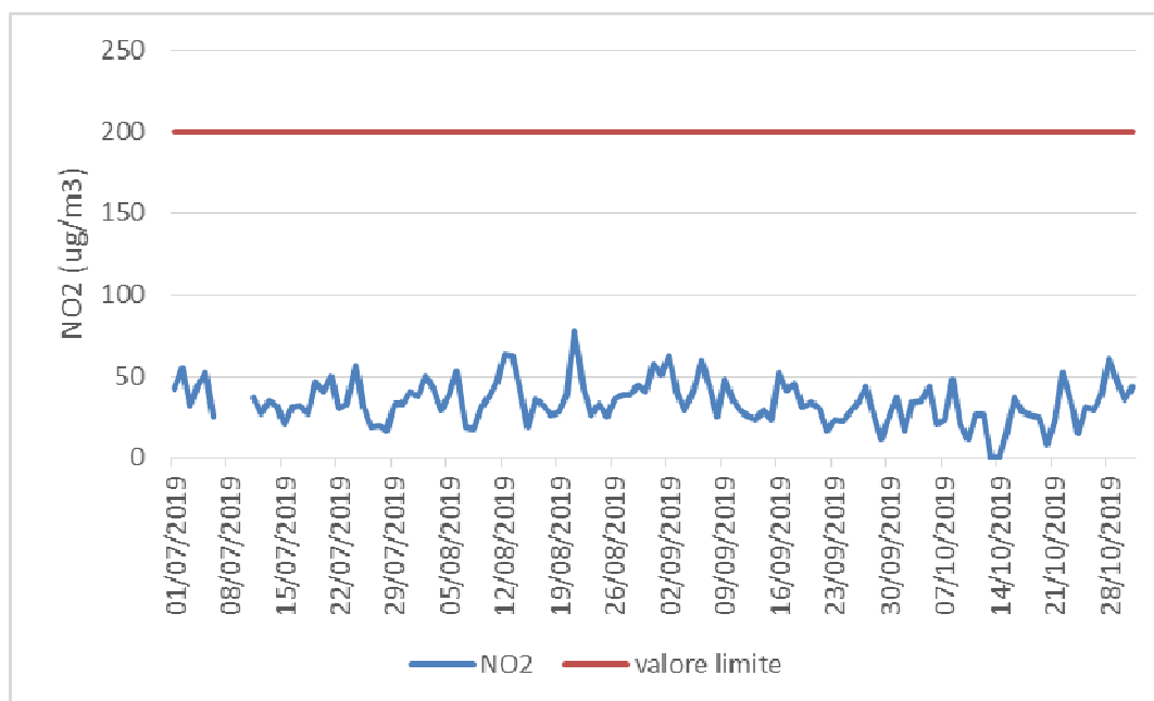
Figura 3b. NO 2 : massimo giornaliero della media oraria
