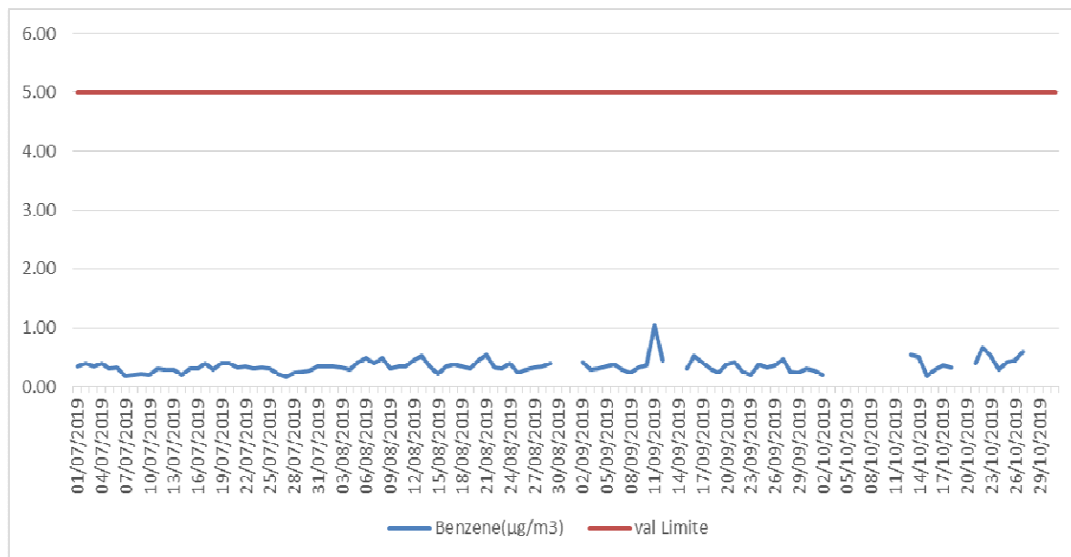
Figura 5a. Benzene: media giornaliera
