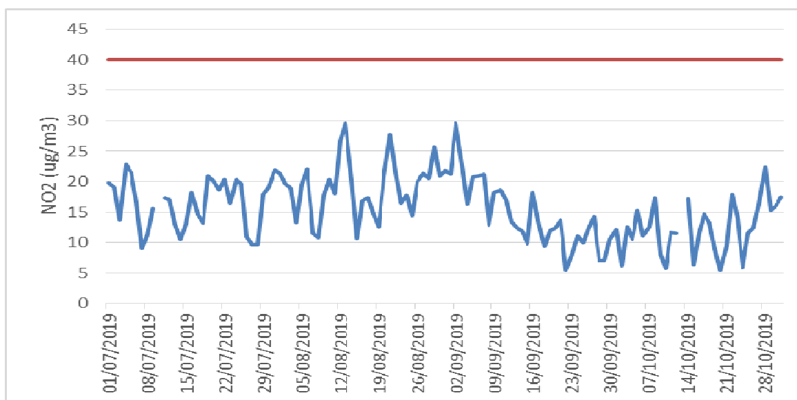
Figura 3a. NO 2 : media giornaliera
