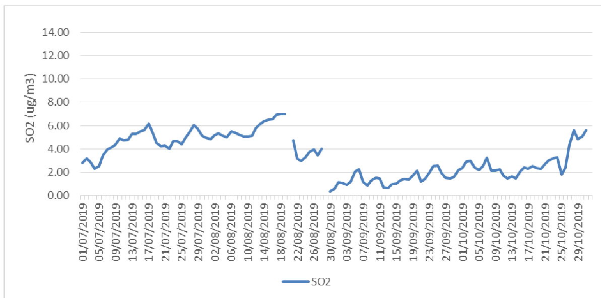
Figura 6. SO 2 : media giornaliera
