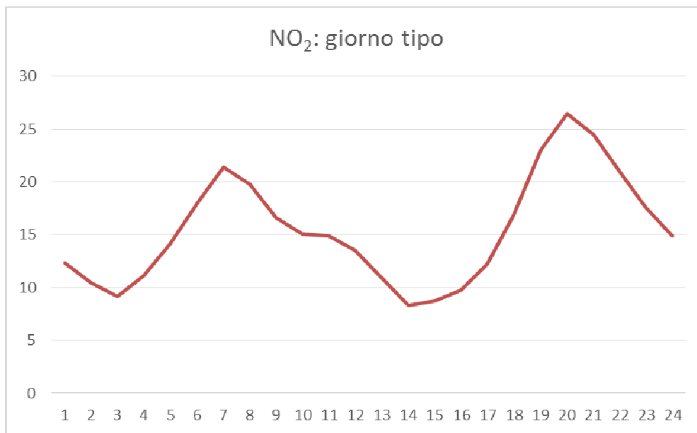
Figura 3c. NO 2 : giorno tipo
