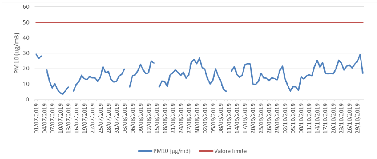
Figura 2. PM10: media giornaliera
