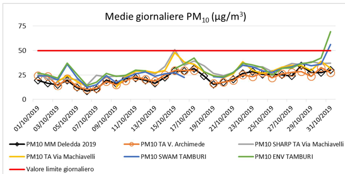
Figura 6. Andamenti giornalieri del PM10 c/o la scuola Deledda e negli altri 3 siti di monitoraggio attivi al quartiere Tamburi nel periodo dal 01/10/2019 al 31/10/2019
