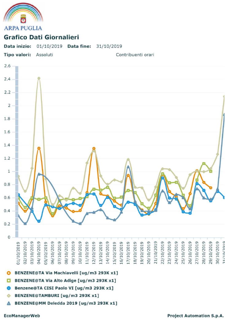
Figura 14. Andamenti medi giornalieri di Benzene a Taranto nel periodo dal 01/10/2019 al 31/10/2019.
