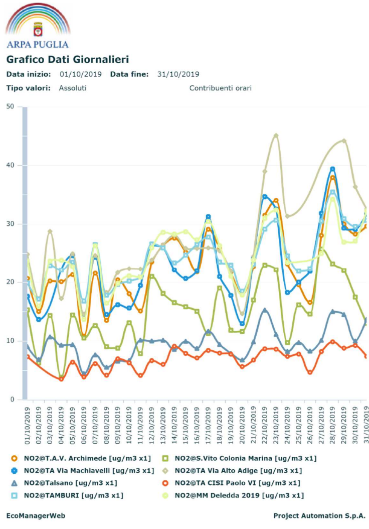
Figura 10. Andamenti medi giornalieri di NO 2 a Taranto nel periodo dal 01/10/2019 al 31/10/2019.
