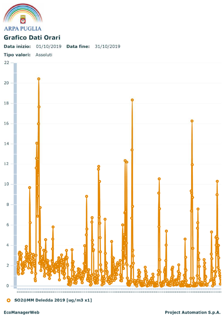
Figura 11. Andamenti orari di SO 2 misurati a Deledda nel periodo dal 01/10/2019 al 31/10/2019.
