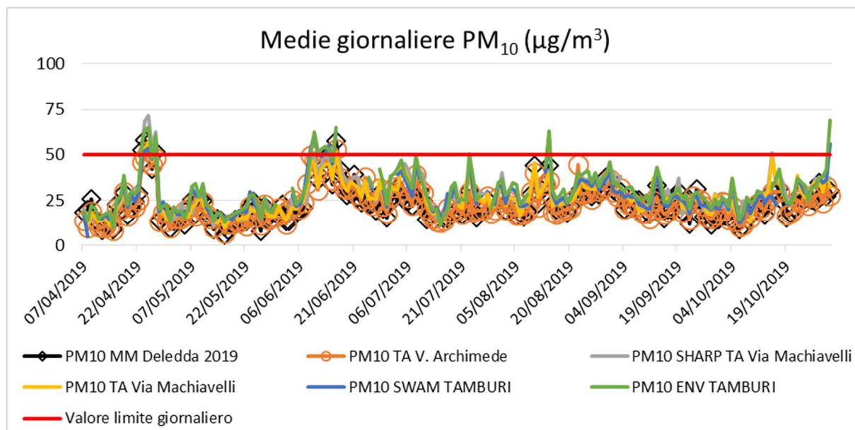
Figura 6a. Andamenti giornalieri del PM10 c/o la scuola Deledda e negli altri 3 siti di monitoraggio attivi al quartiere Tamburi nel periodo dal 07/04/2019 al 31/10/2019
