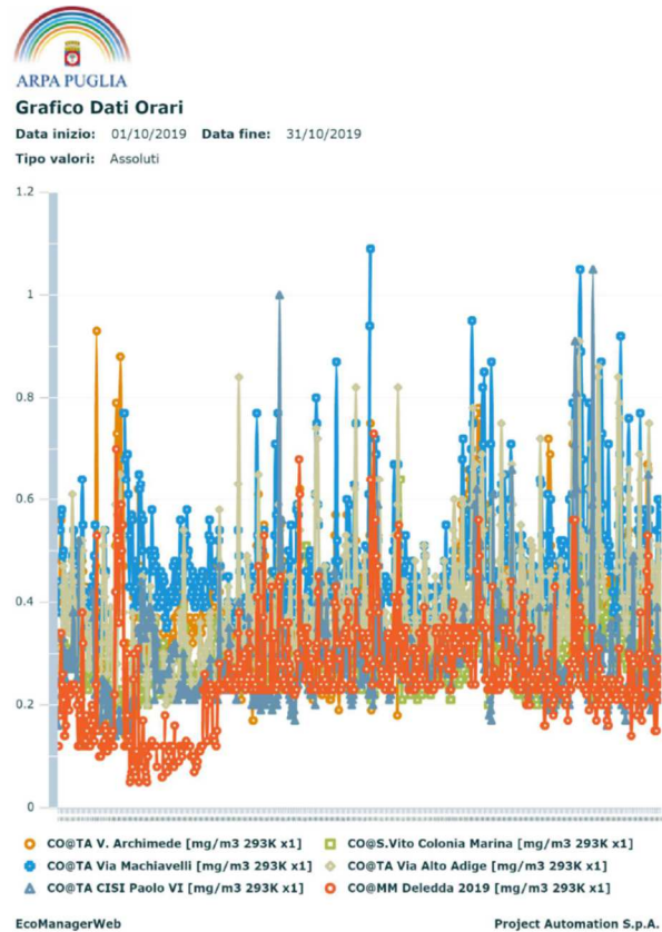
Figura 13. Andamenti orari di CO a Taranto nel periodo dal 01/10/2019 al 31/10/2019.
