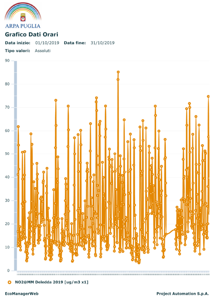
Figura 9. Andamenti orari dell'NO 2 misurato c/o Deledda dal 01/10/2019 al 31/10/2019.
