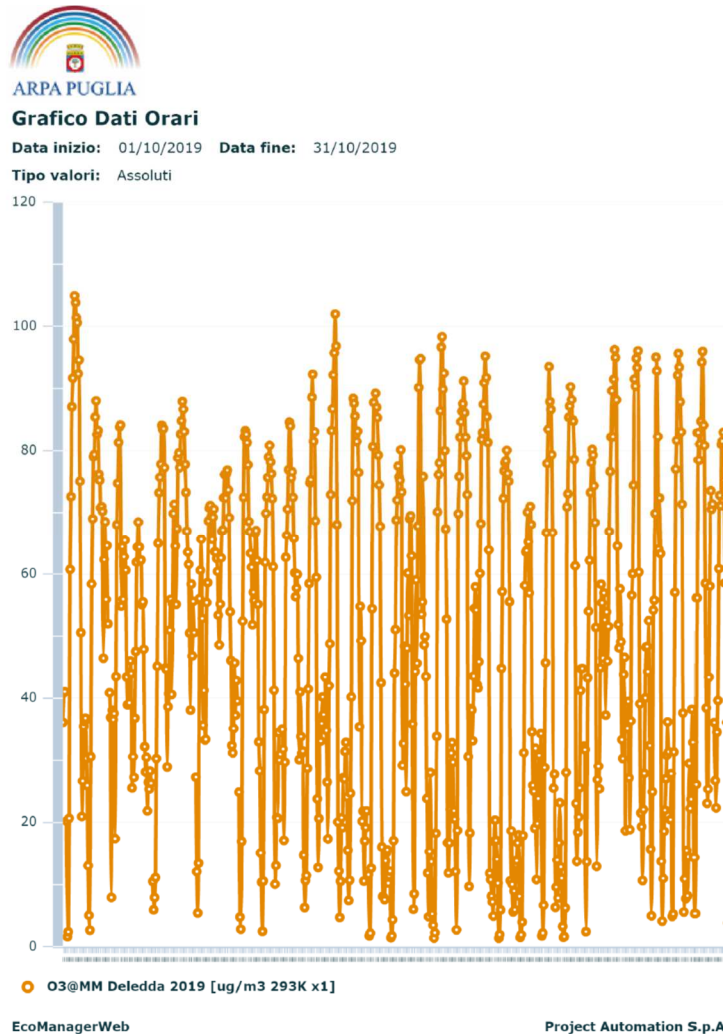
Figura 8. Andamenti orari dell'Ozono misurato c/o la Scuola Deledda nel periodo dal 01/10/2019 al 31/10/2019.
