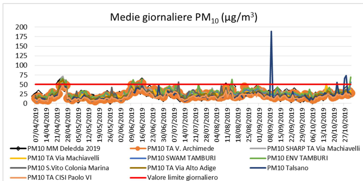
Figura 7a. Andamenti giornalieri del PM 10 misurato a Taranto nel periodo dal 07/04/2019 al 31/10/2019
