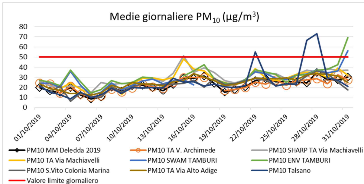
Figura 7. Andamenti giornalieri del PM 10 misurato a Taranto nel periodo dal 01/10/2019 al 31/10/2019
