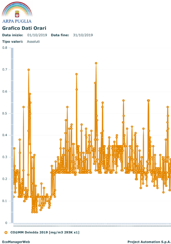
Figura 12. Andamenti orari di CO a Deledda nel periodo dal 01/10/2019 al 31/10/2019.
