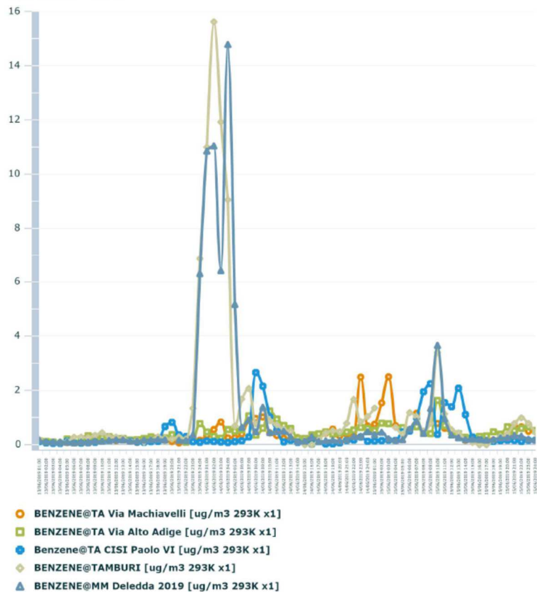
Figura 14 c - Andamenti orari di Benzene nelle stazioni di Taranto dal 13/06/2019 al 15/06/2019
