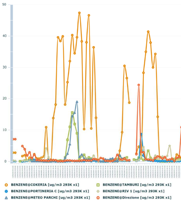
Figura 14 a - Andamenti orari di Benzene rete AMI dal 13/06/2019 al 15/06/2019
