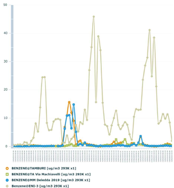
Figura 14 b - Andamenti orari di Benzene nelle stazioni di Tamburi-Taranto e in ENI3 nel periodo dal 13/06/2019 al 15/06/2019
