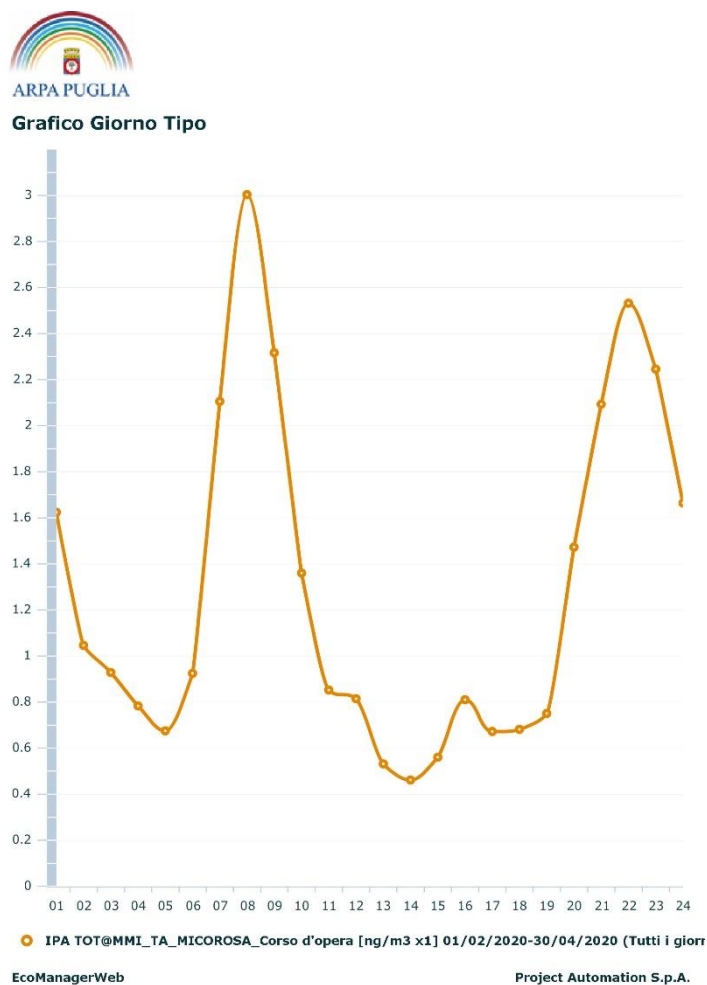
Figura 11: Grafico del giorno tipo per gli idrocarburi policiclici aromatici totali.
