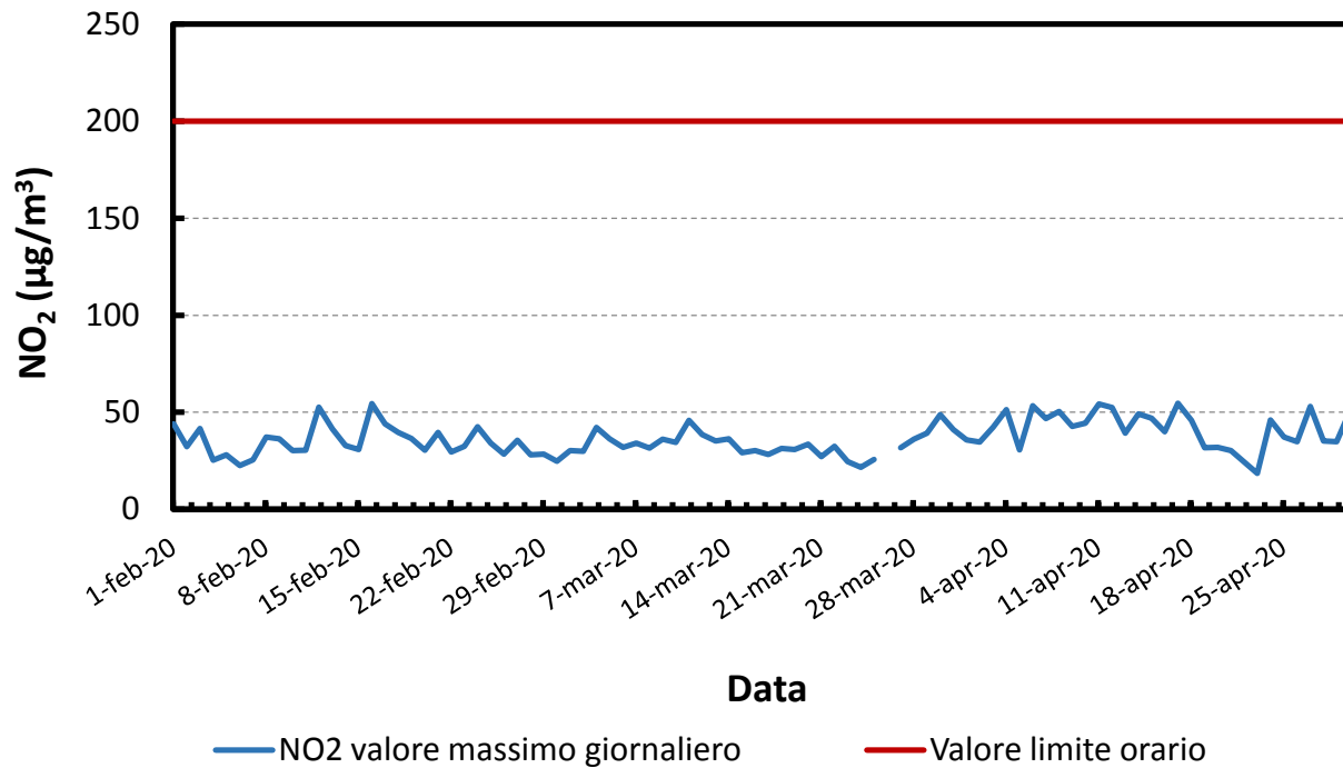
Figura 17: Andamento della concentrazione massima oraria giornaliera del biossido di azoto
