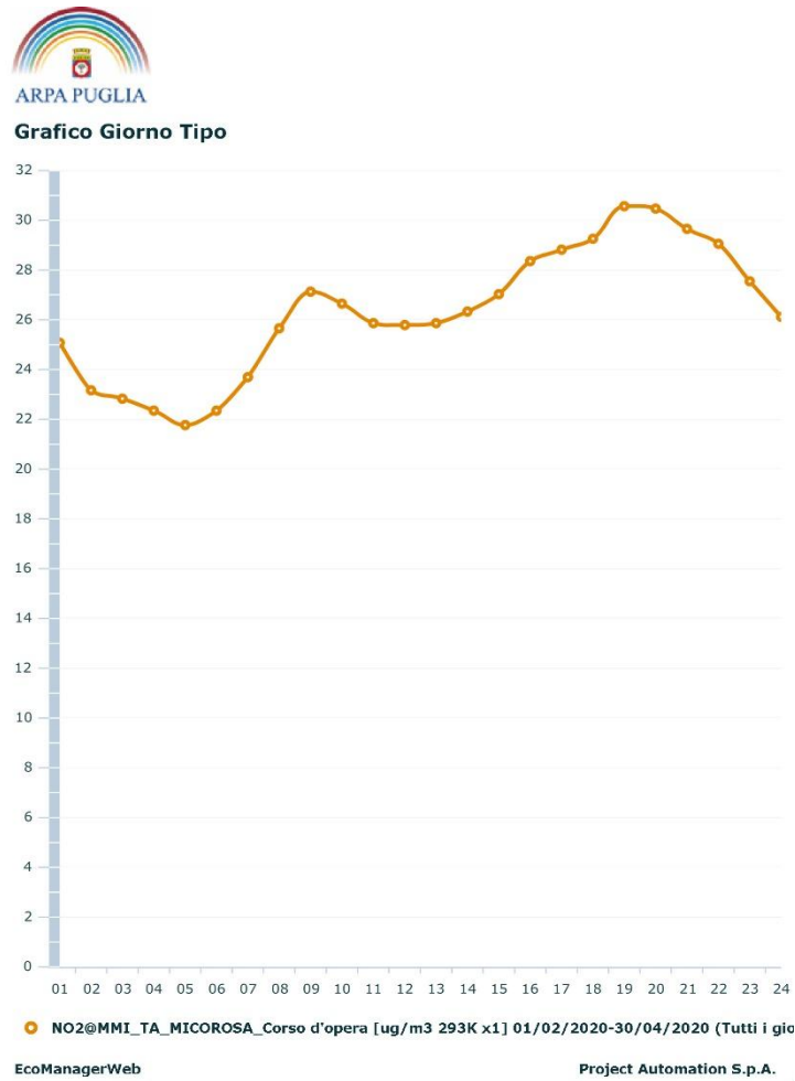
Figura 5: Grafico del giorno tipo per l'inquinante NO 2 .
