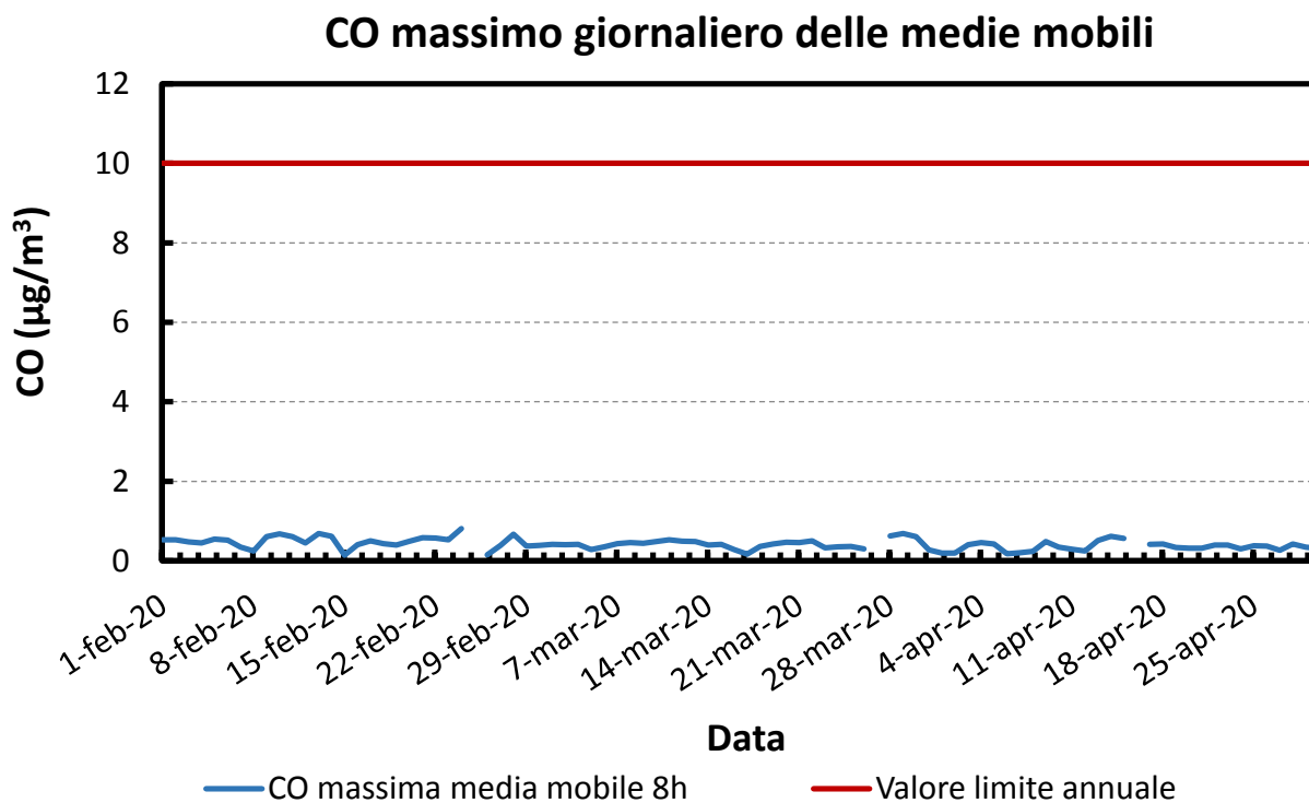
Figura 21: Andamento della media mobile su 8 ore massima giornaliera del monossido di carbonio
