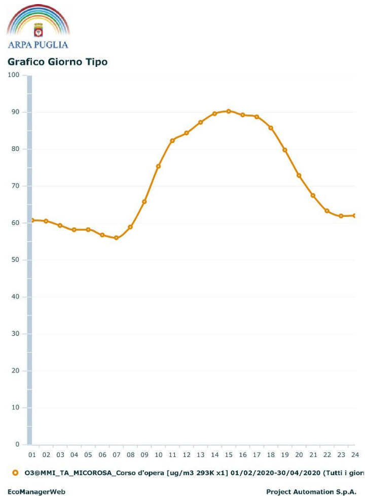
Figura 7: Grafico del giorno tipo per l'inquinante O 3 .
