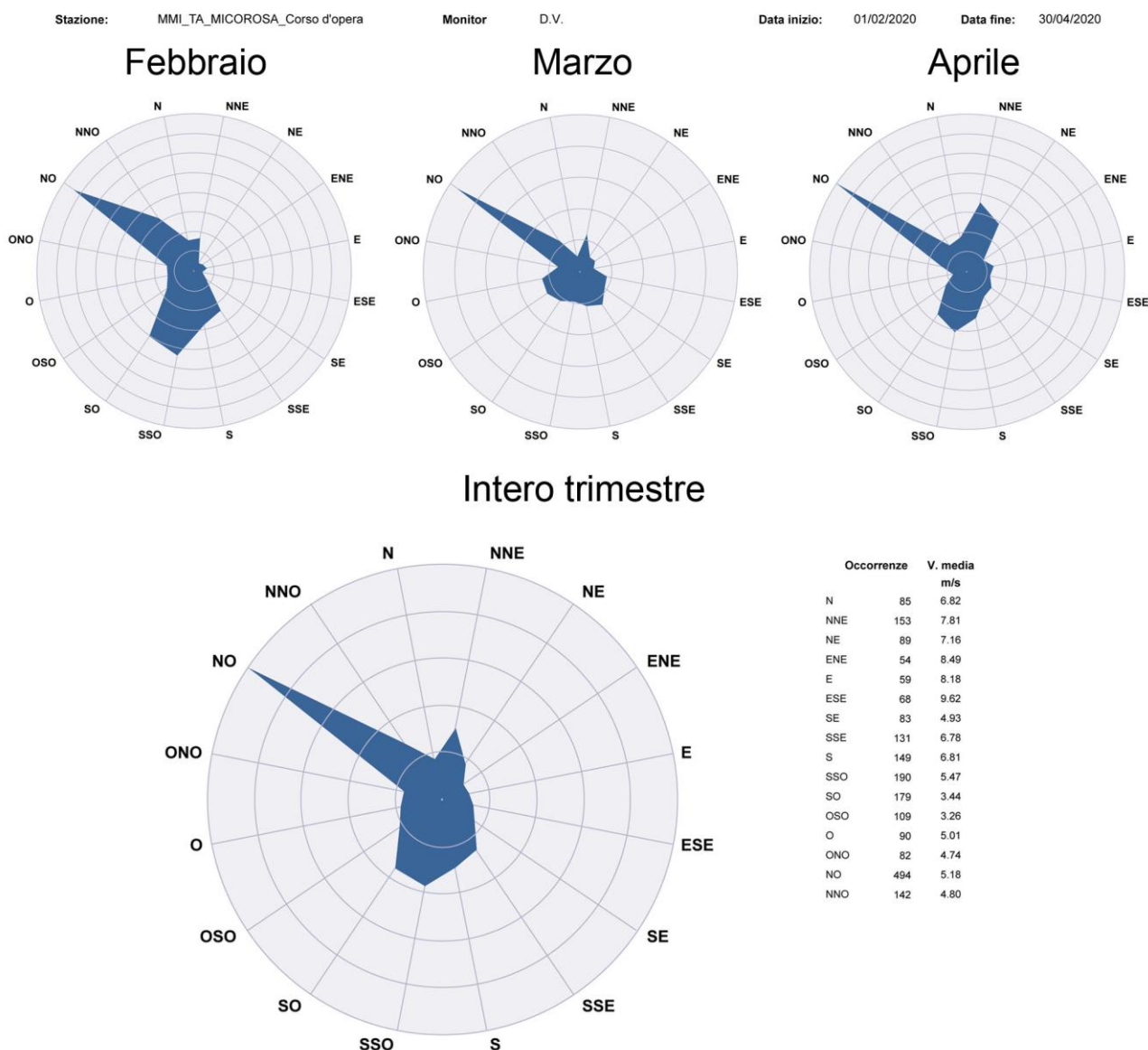
Figura 3: Rose dei venti per i mesi di febbraio, marzo e aprile e per l'intero periodo di monitoraggio, corredato dalla tabella complessiva delle occorrenze.
