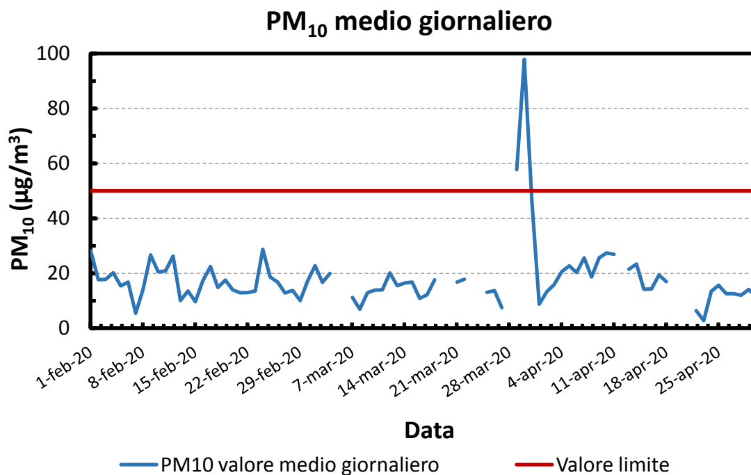
Figura 12: Andamento giornaliero del PM 10 .
