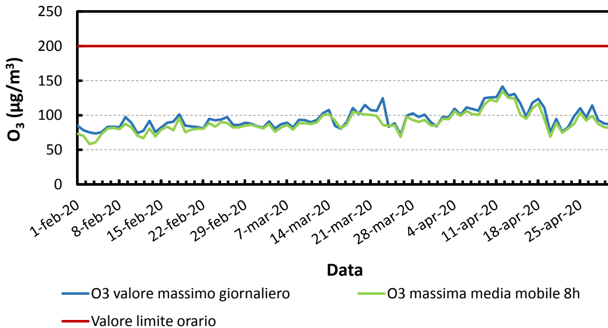
Figura 15: Andamento giornaliero del valore massimo e della massima media mobile misurata sulle 8 ore per l’ozono.
