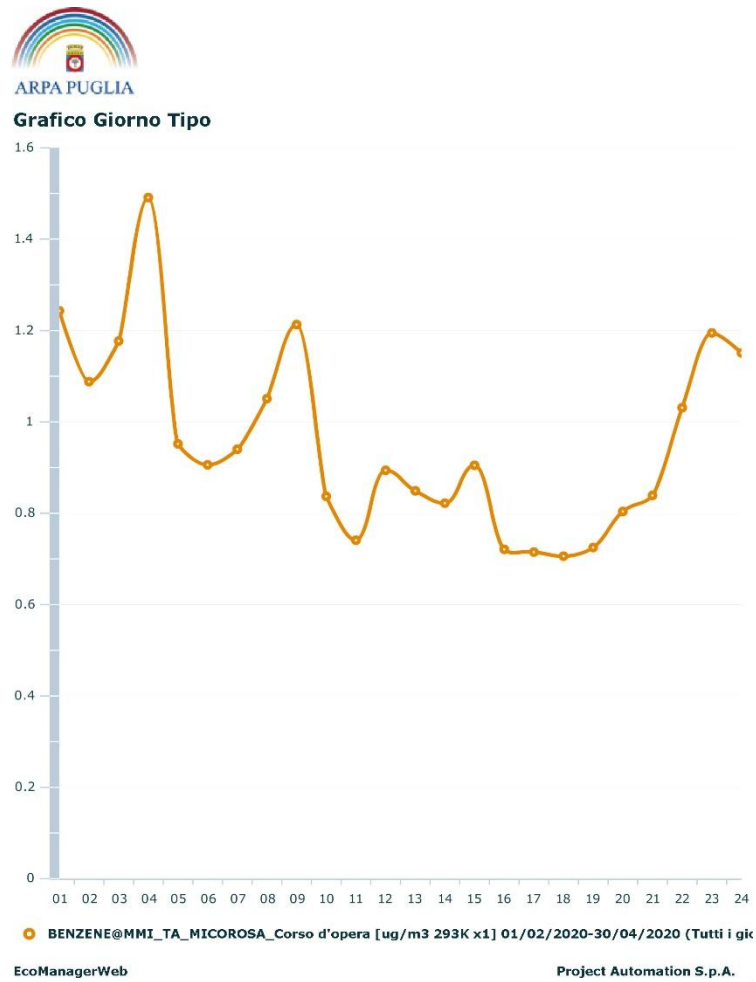
Figura 8: Grafico del giorno tipo per l'inquinante benzene.
