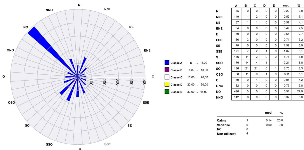
Figura 23: Rosa dell'inquinamento per gli idrocarburi policiclici aromatici.
