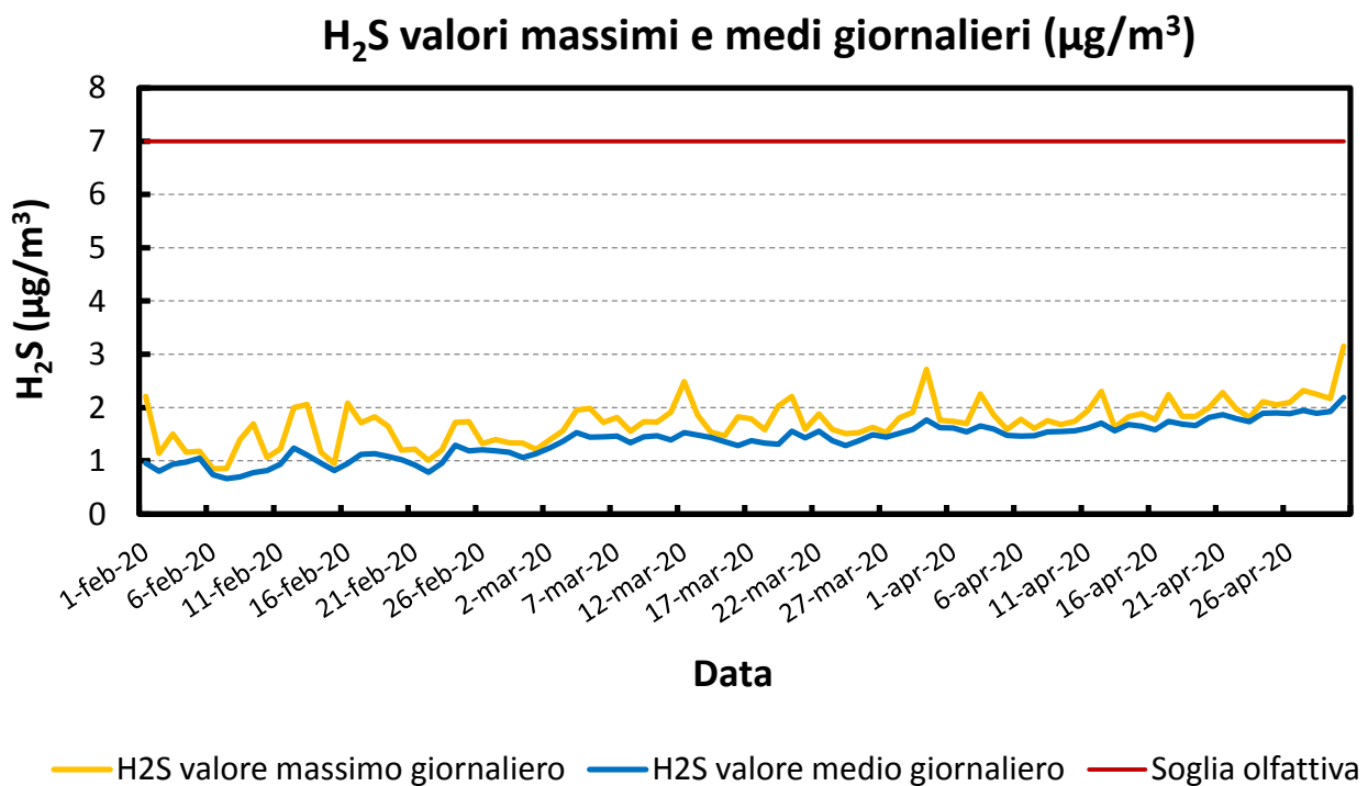
Figura 24: Andamento della concentrazione media e massima giornaliera di acido solfidrico
