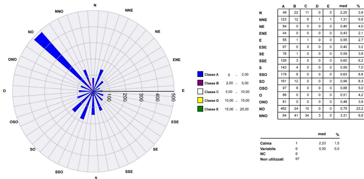
Figura 23: Rosa dell'inquinamento per l'inquinante benzene.
