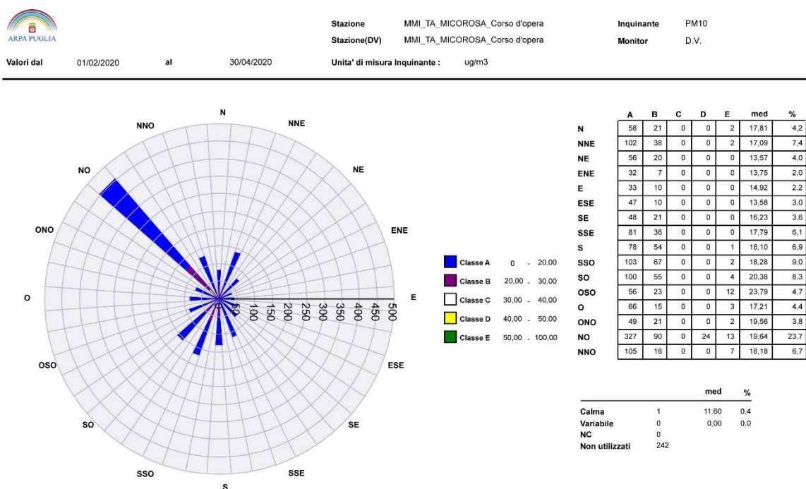
Figura 23: Rosa dell'inquinamento per il PM 10 .
