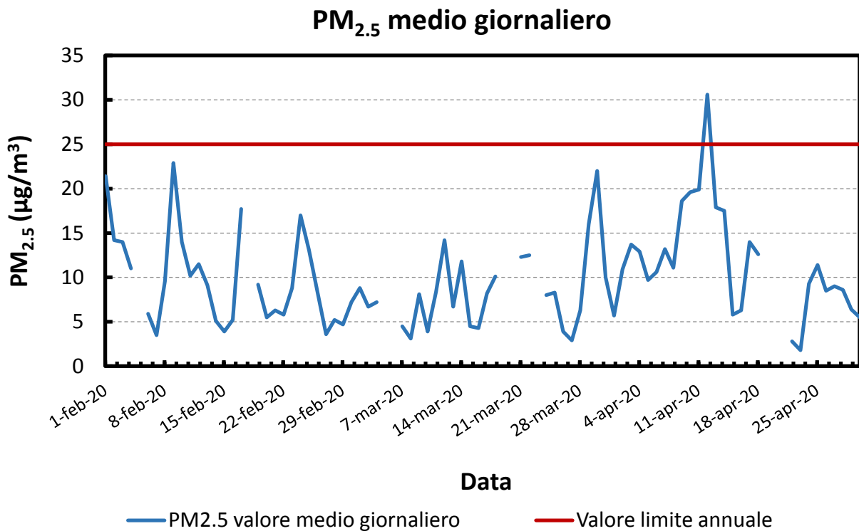
Figura 14: Andamento giornaliero del PM 2.5 .
