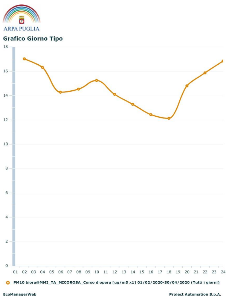
Figura 4: Grafico del giorno tipo di PM10 ottenuto con analizzatore biorario.
