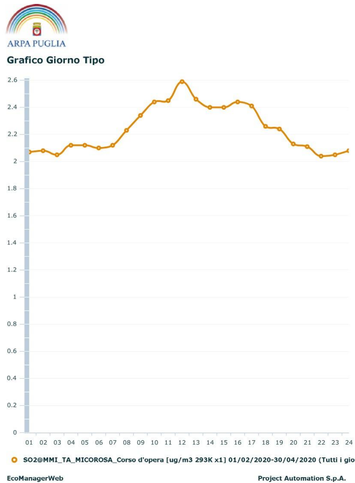
Figura 10: Grafico del giorno tipo per l'inquinante SO 2 .
