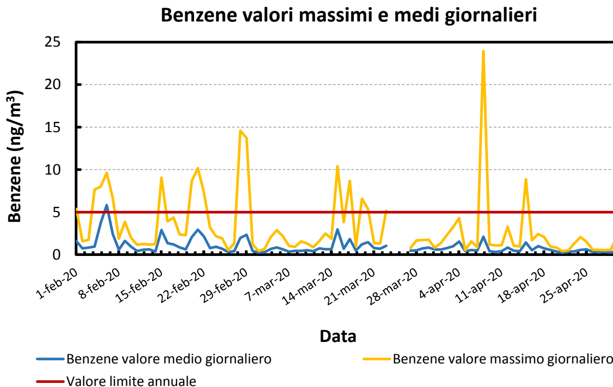
Figura 22: Andamento della concentrazione media e massima giornaliera del benzene
