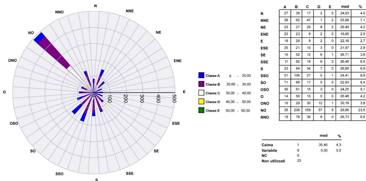
Figura 48: Rosa dell'inquinamento per l'inquinante biossido di azoto.
