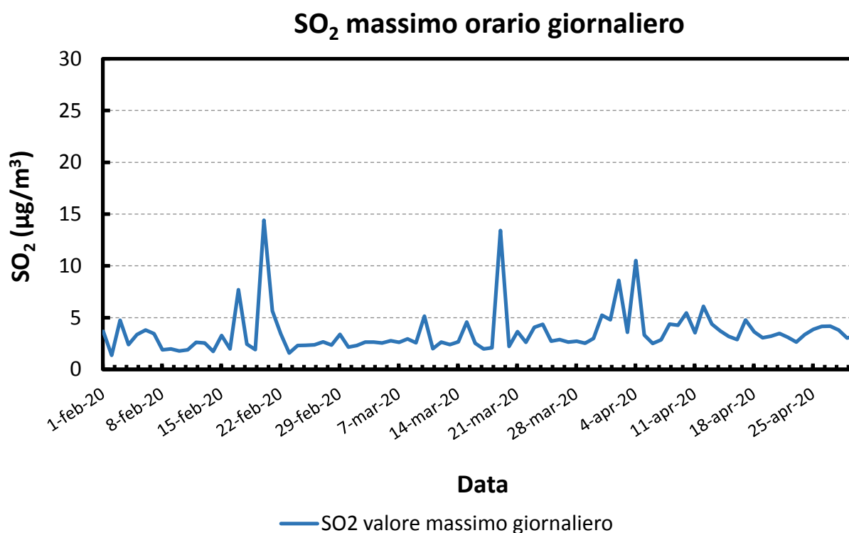
Figura 19: Andamento della concentrazione massima oraria giornaliera del biossido di zolfo
