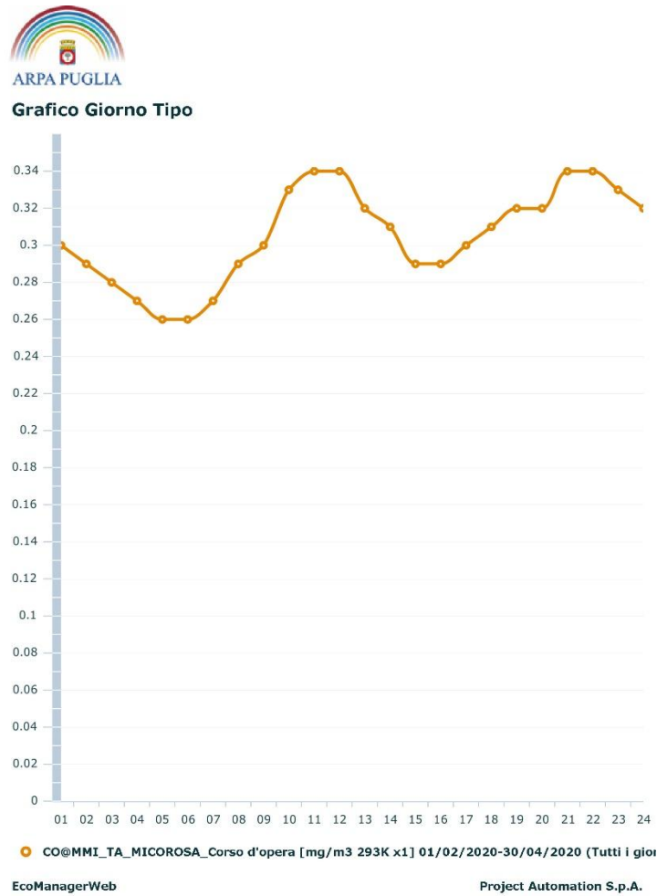
Figura 6: Grafico del giorno tipo per l'inquinante CO.
