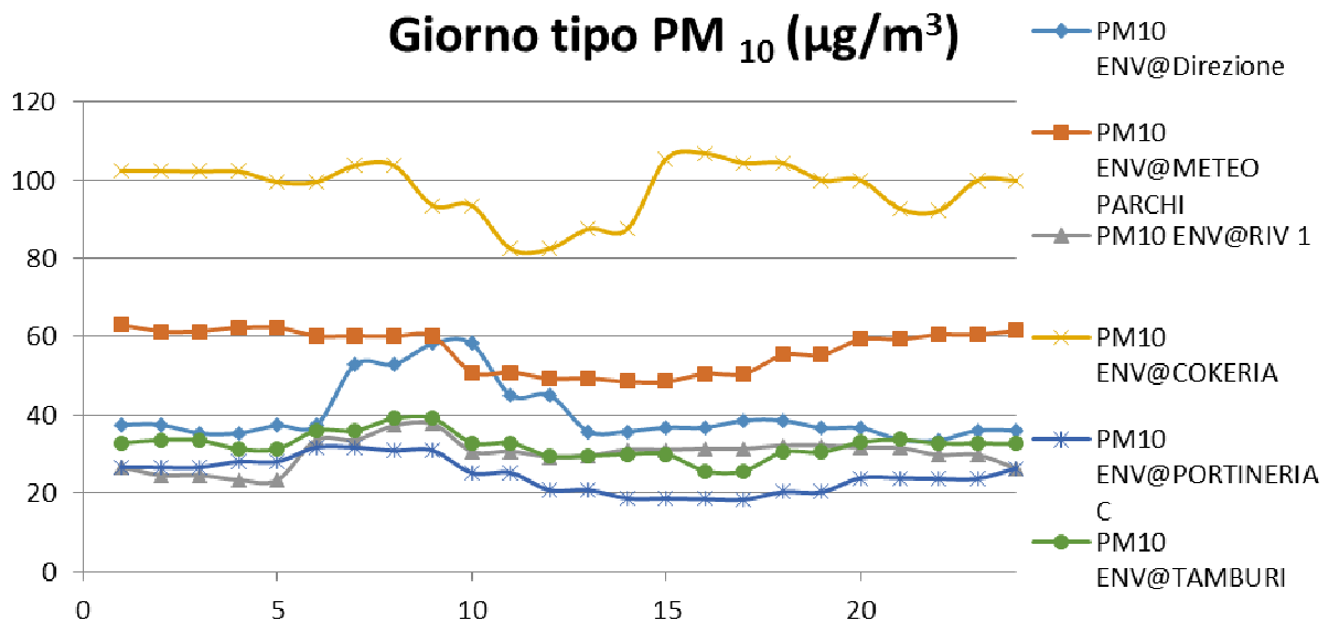
Fig.4 - Giorno tipo delle concentrazioni di PM 10
