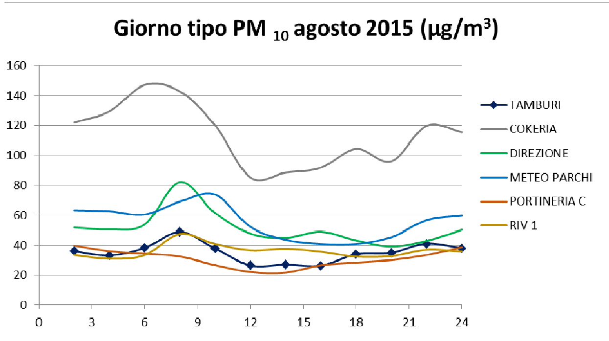
Fig.6 - Giorno tipo delle concentrazioni di PM 10
