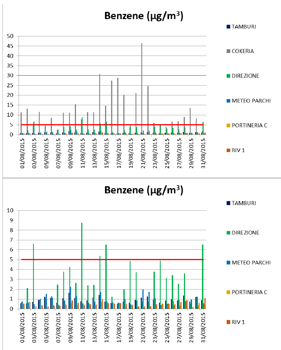
Fig.8 - Livelli di concentrazione di Benzene
