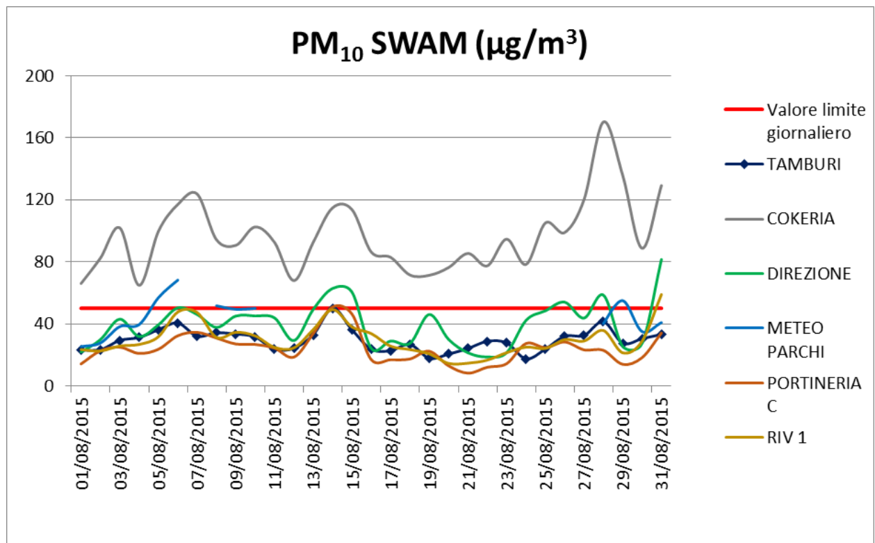
Fig.3 - Livelli di concentrazione di PM 10 (SWAM) in \mu\text{g}/\text{m}^3
