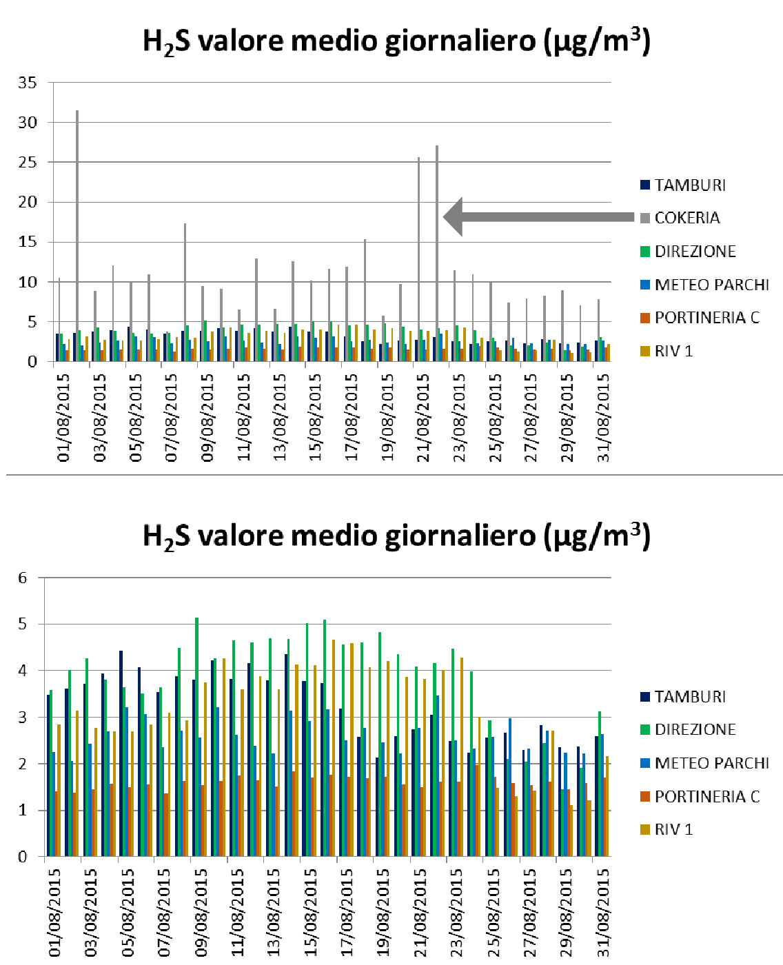
Fig.2 - Livelli di concentrazione di H 2 S in \mu\text{g}/\text{m}^3
