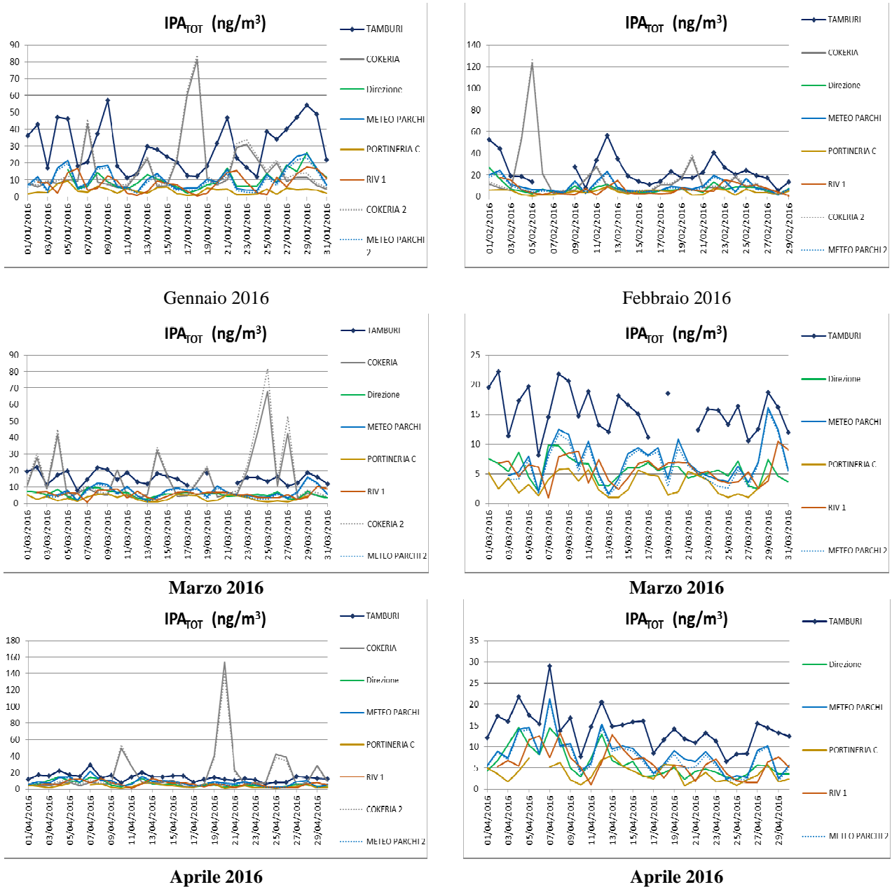
Fig. 14 - Livelli di concentrazione di IPA TOT
