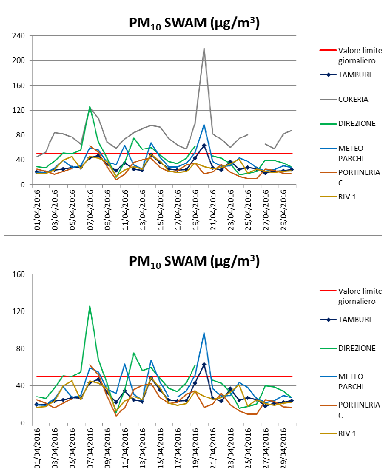
Fig. 3 - Livelli di concentrazione di PM 10 (SWAM) in µg/m 3
