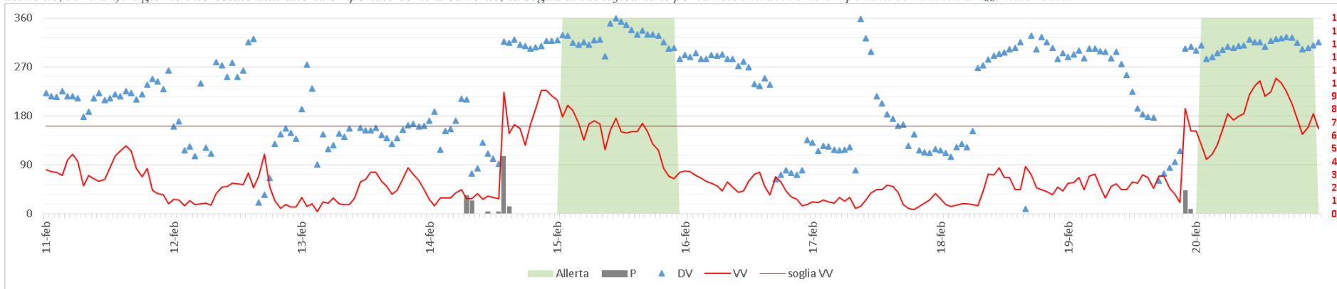
Figura 5: Velocità del vento (linea rossa, asse a destra, in m/s), direzione del vento (triangoli blu, asse a sinistra), precipitazione cumulata oraria (istogramma in grigio, stesso asse a destra della velocità del vento, in mm/h). Il giorno interessato dall'allerta è riportato come area verde; la soglia di identificazione per la velocità del vento è riportata come linea orizzontale rossa.
