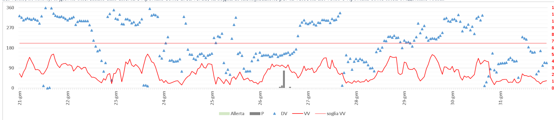
Figura 3: Velocità del vento (linea rossa, asse a destra, in m/s), direzione del vento (triangoli blu, asse a sinistra), precipitazione cumulata oraria (istogramma in grigio, stesso asse a destra della velocità del vento, in mm/h). Il giorno interessato dall'allerta è riportato come area verde; la soglia di identificazione per la velocità del vento è riportata come linea orizzontale rossa.
