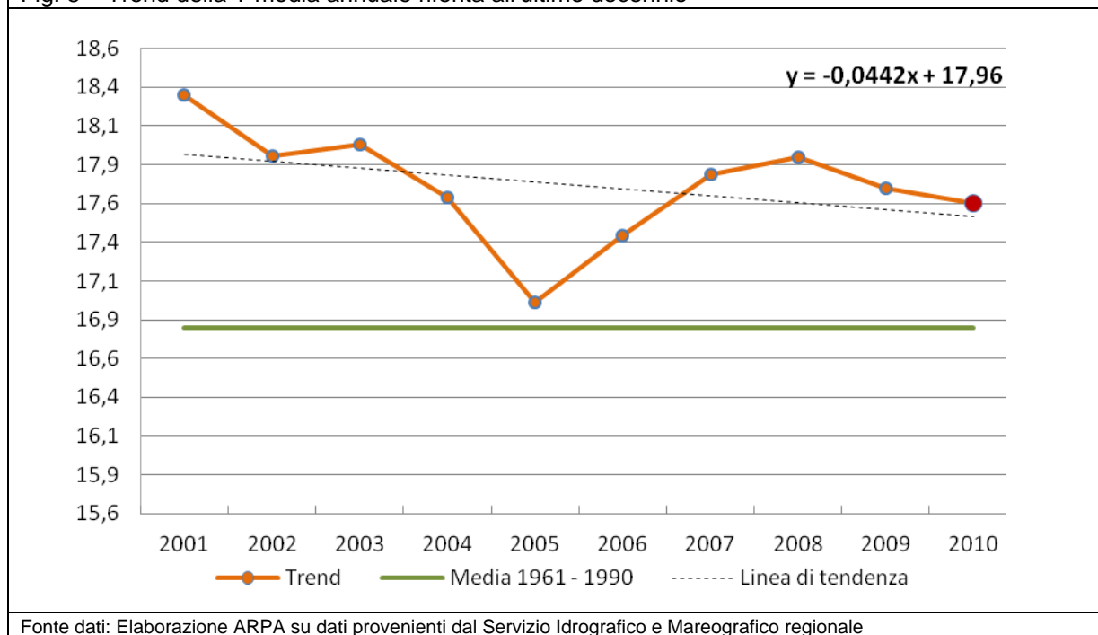
Fig. 5 – Trend della T media annuale riferita all'ultimo decennio
