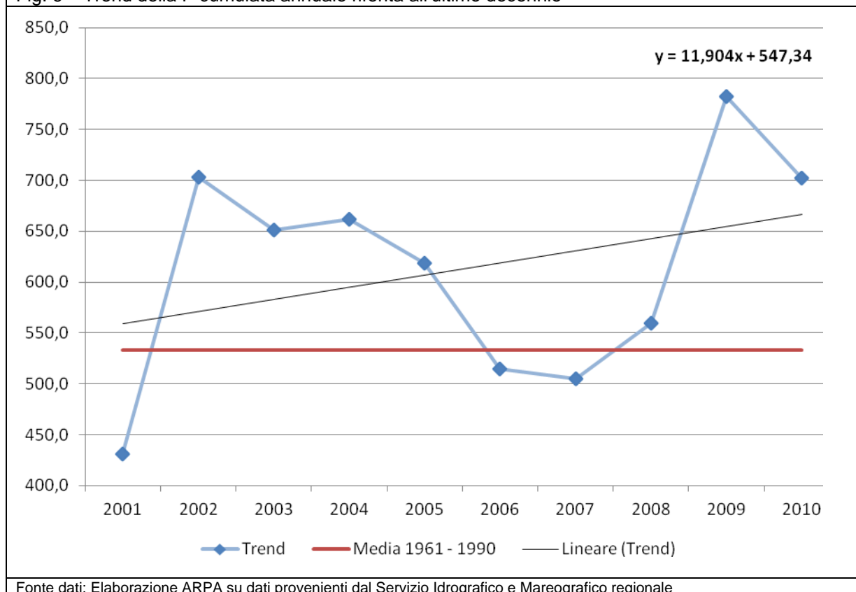
Fig. 6 – Trend della P cumulata annuale riferita all'ultimo decennio
