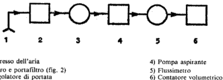
Schema B - Prelievo di campioni di inquinanti per filtrazione dell'aria
